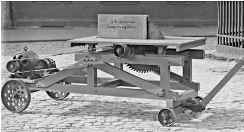
Alte Kreissäge 30er Jahre mit Keilriemenantrieb.
